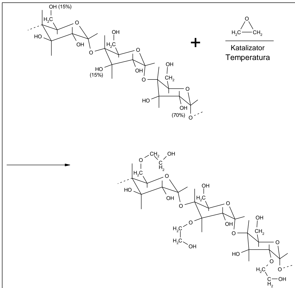
Ryc. 4. Synteza i budowa HES
